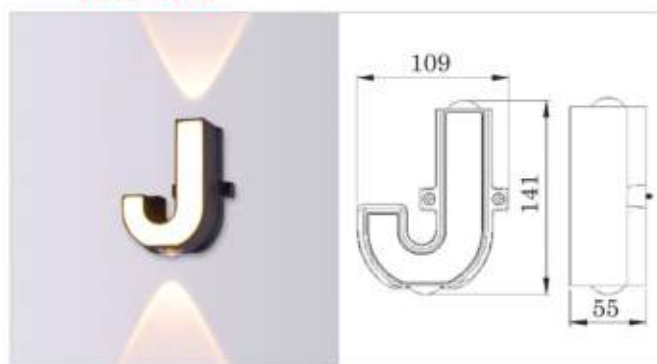
CHỮ J LED 8W - 3000K 780.000đ
