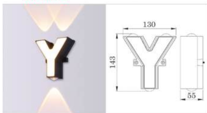
CHỮ Y LED 11W - 3000K 780.000đ
