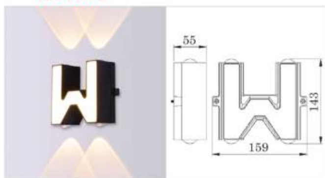
CHỮ W LED 12W - 3000K 780.000đ
