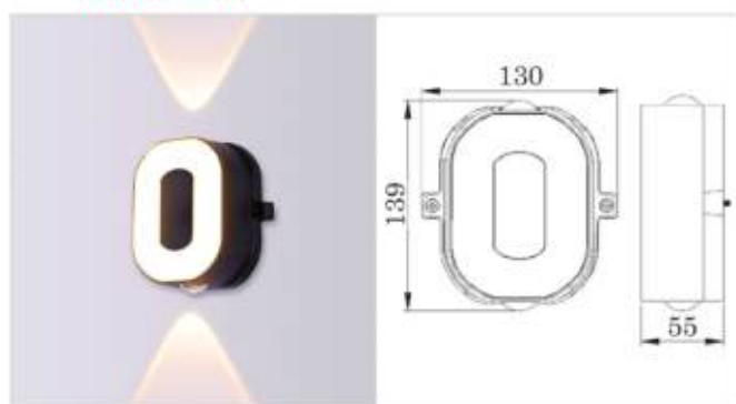
CHỮ O LED 10W - 3000K 780.000đ
