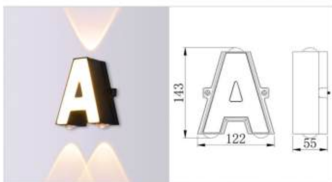
CHỮ A LED 11W - 3000K 780.000đ
