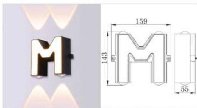
CHỮ M LED 12W - 3000K 780.000đ
