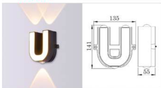
CHỮ U LED 11W - 3000K 780.000đ
