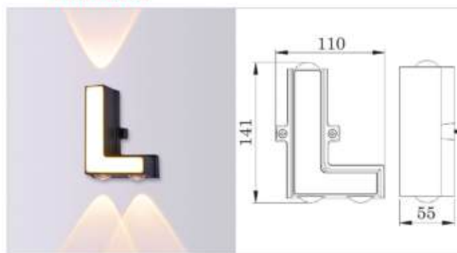
CHỮ L LED 8W - 3000K 780.000đ
