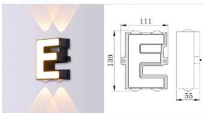
CHỮ E LED 11W - 3000K 780.000đ
